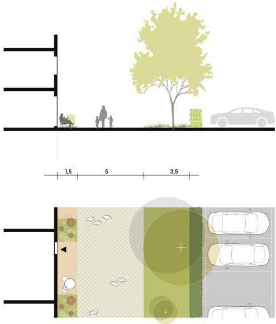
Profiel tussenstraat
