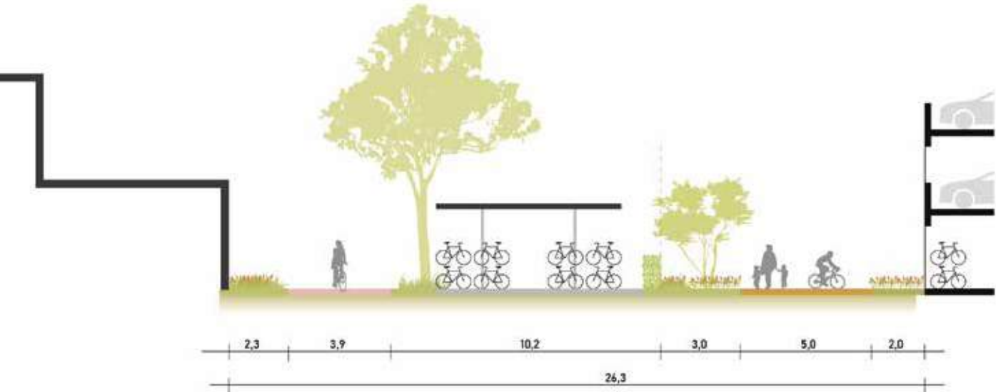
Profiel Bonepadsweg en noordzijde Kop van de Boulevard
